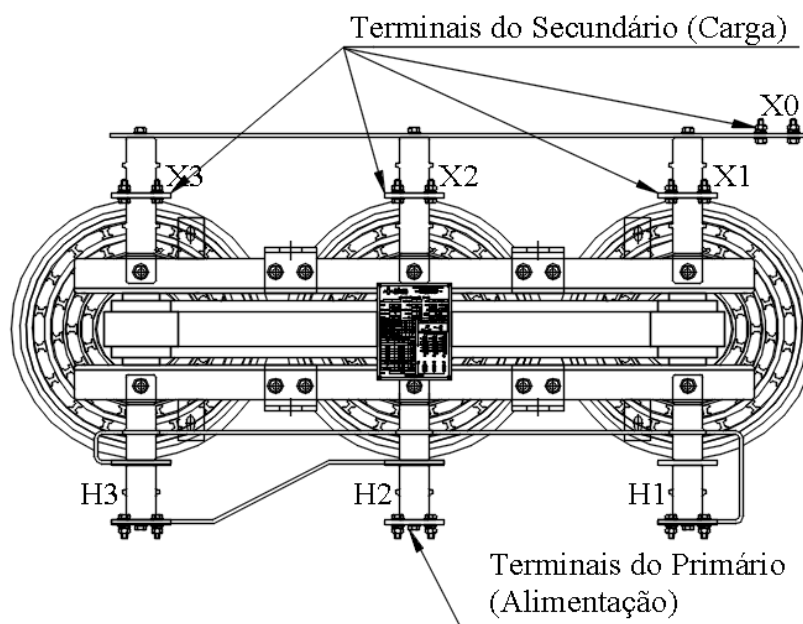
Figura 9 – Identificação de Terminais – Vista Superior Transformador Trifásico
