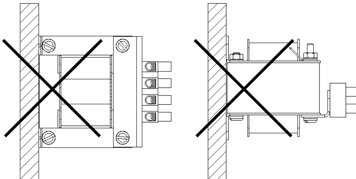
Figura 7 – Posições Proibidas para Montagem
