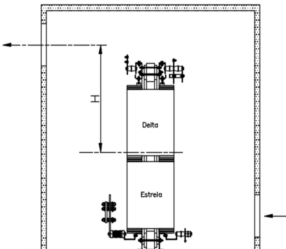
Figura 8 – Ventilação Adequada
