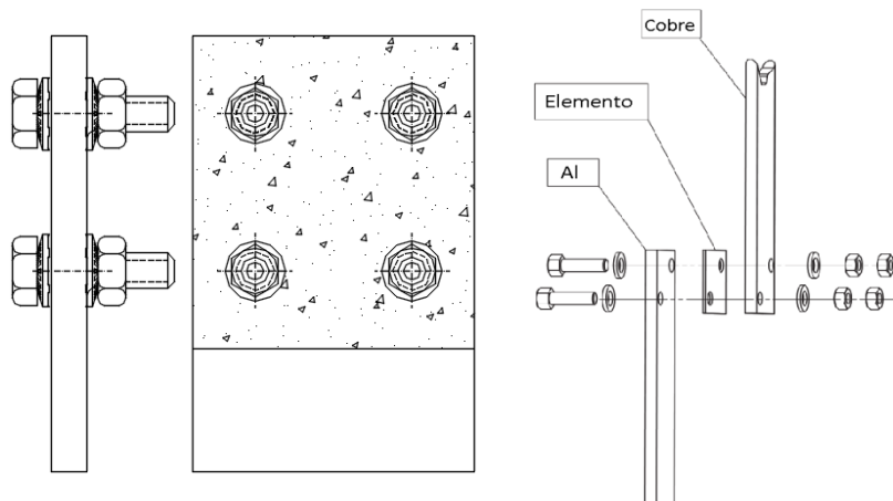
Figura 10 - Tipo de terminais disponibilizados para conexão do primário/secundário do transformador com elemento bimetálico
