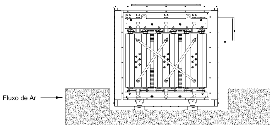
Figura 8 – Fluxo de ar obstruído
