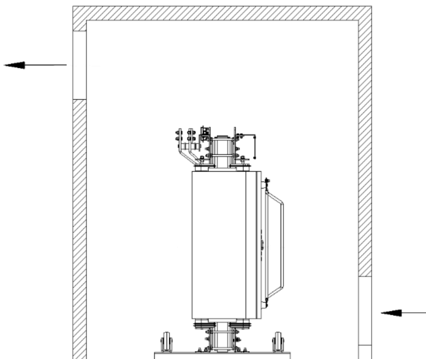
Figura 6 – Entrada de ar para ventilação natural
