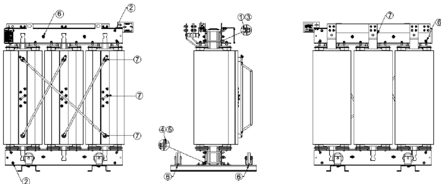
Figura 3: Reaperto das conexões
