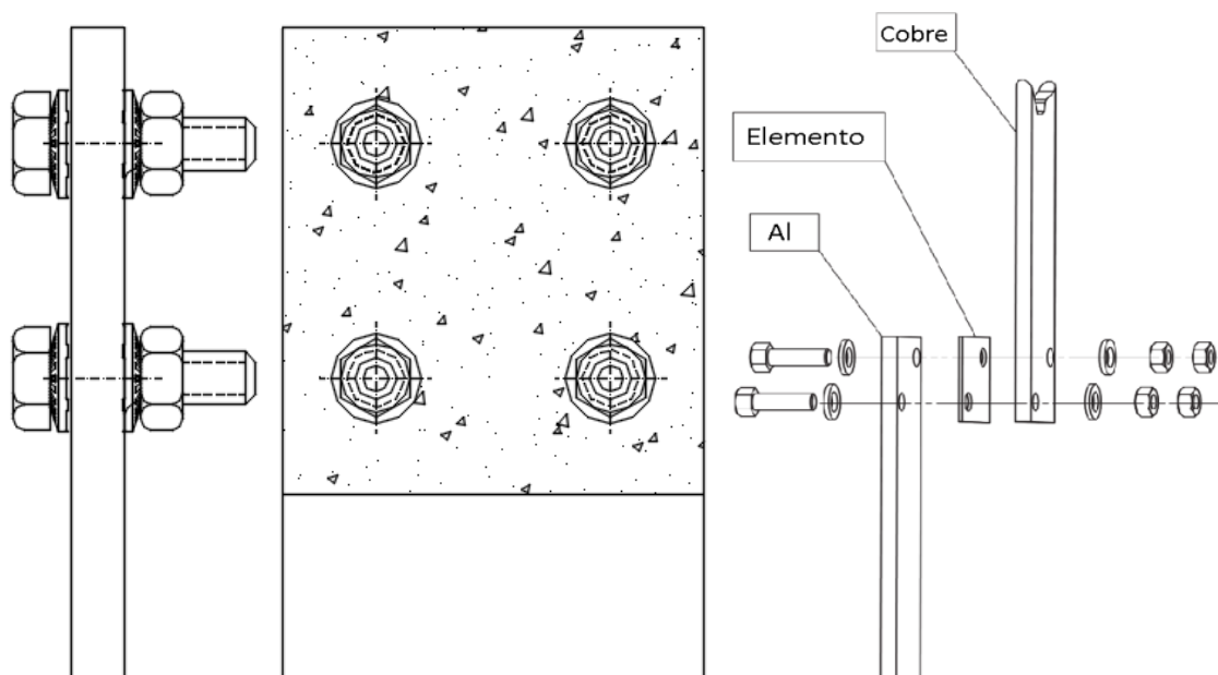
Figura 4 - Tipo de terminais disponibilizados para conexão dos terminais do transformador com elemento bimetálico
